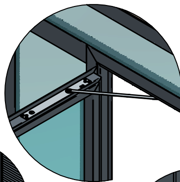
DETAIL B ferme-porte encastré
