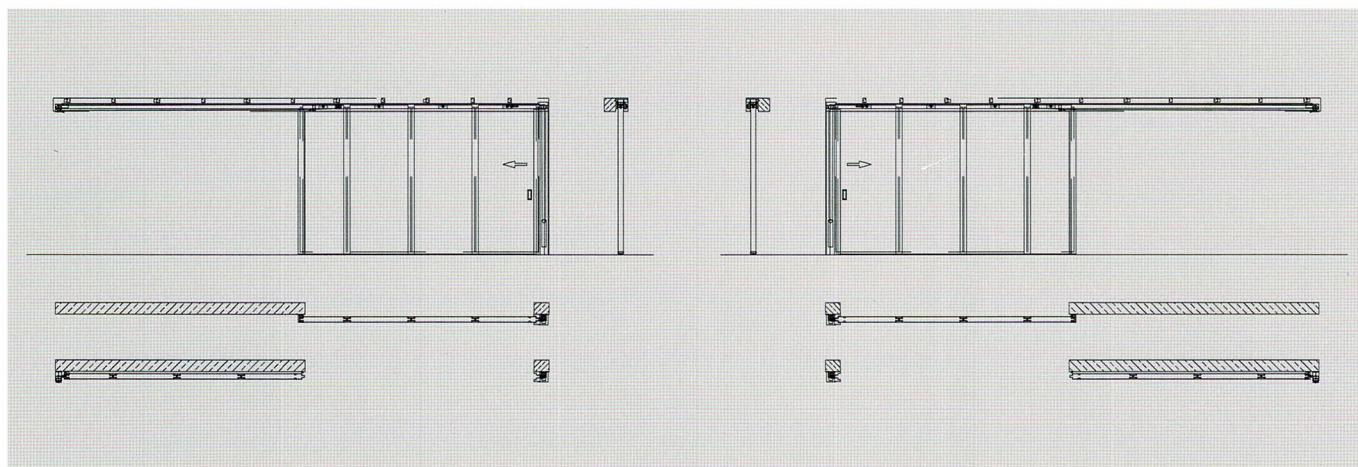
a) porte coulissante avec le sens d'ouverture vers la gauche
