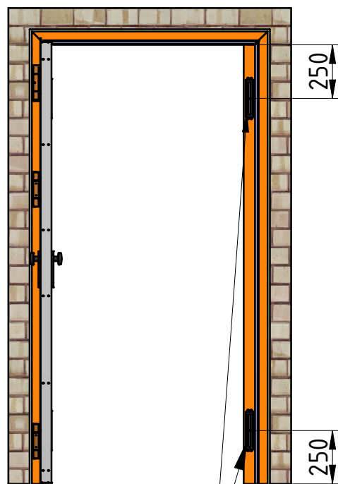
ventouses électromagnétiques encastrées 300 kg
