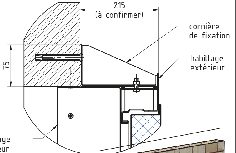
DÉTAIL A
