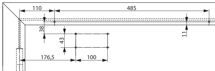
2 - Montage sur la porte côté opposé aux charnières
